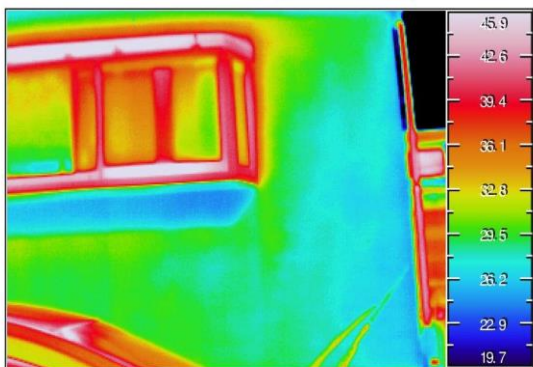
サーモカメラによる、断熱補強の必要な場所と筋交いの有無を確認しました。
