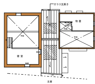
改修後 2階平面図
