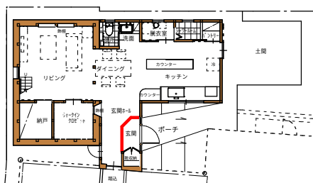
改修後 1階平面図
