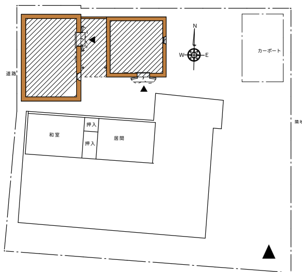
改修前 配置図・平面図
