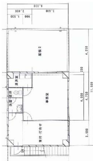
2 階平面図
