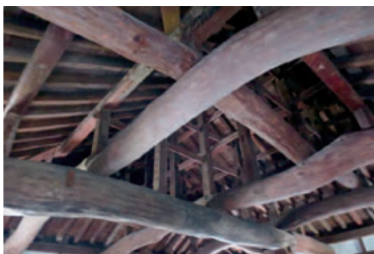
特徴ある梁
